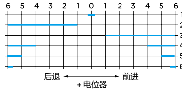
CD方向电气原理图
