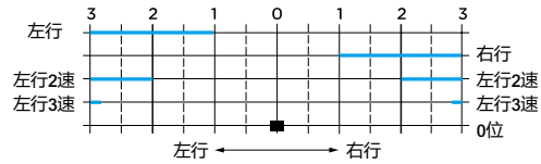
CD方向触点闭合图
