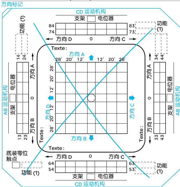
图 1：每运动机构 4 副触点 (顶视图)
