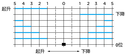
AB方向触点闭合图
